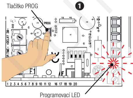
Programovací LED
